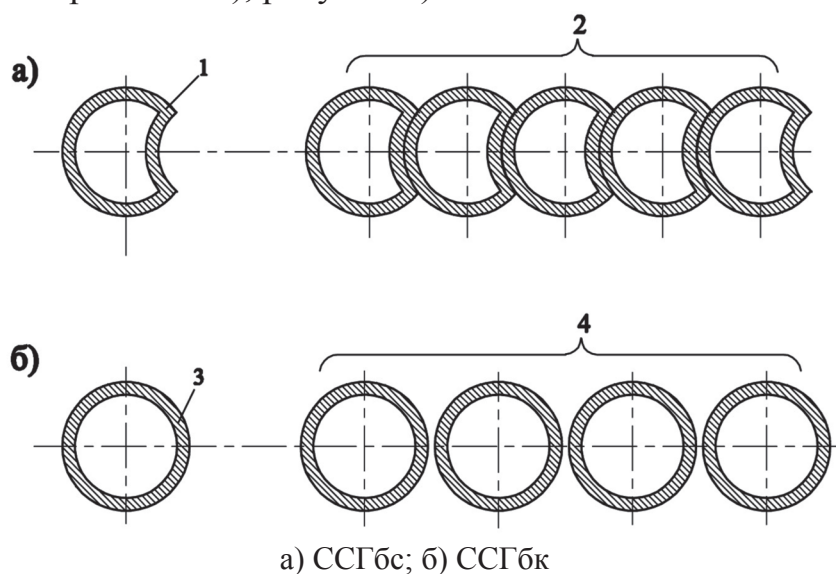
а) ССГбс; б) ССГбк 1 – сечение обсадной трубы ССГбс; 2 – захватка из труб ССГбс; 3 – сечение обсадной трубы ССГбк; 4 – захватка из труб ССГбк
