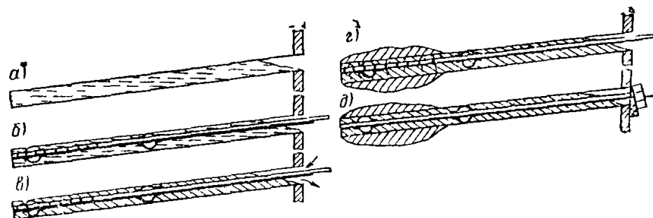
Рис. 3. Технология устройства анкера с иньекционной трубкой
