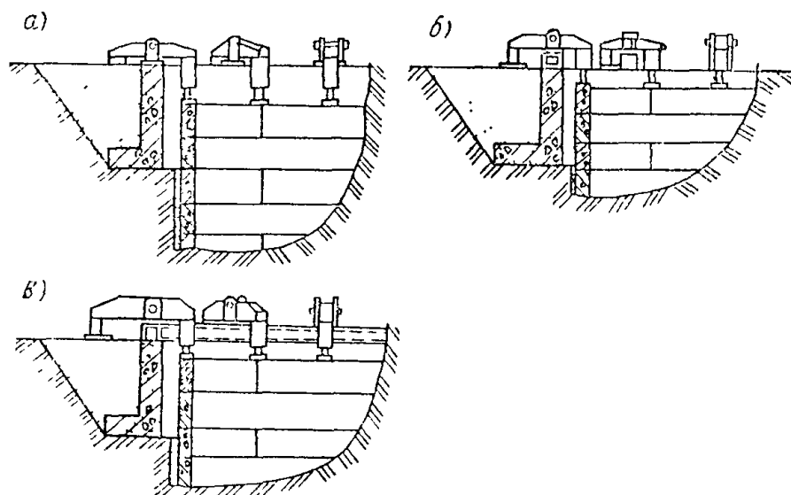
Рис. 109. Устройство для задавливания опускного колодца
