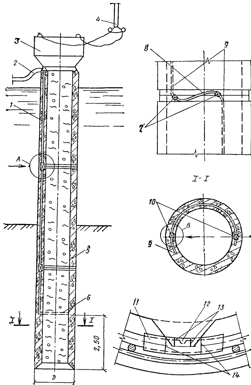
Рис. 2. Схема вибропогружения сваи-оболочки с устройством воздухоподачи
