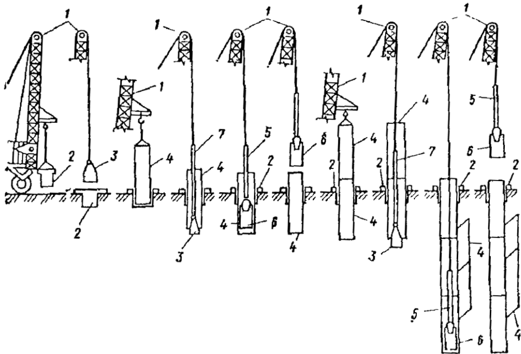
Рис. 3. Устройство скважин станком ударно-канатного бурения
