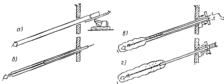
Рис. 1. Технология устройства анкера с теряемым башмаком
