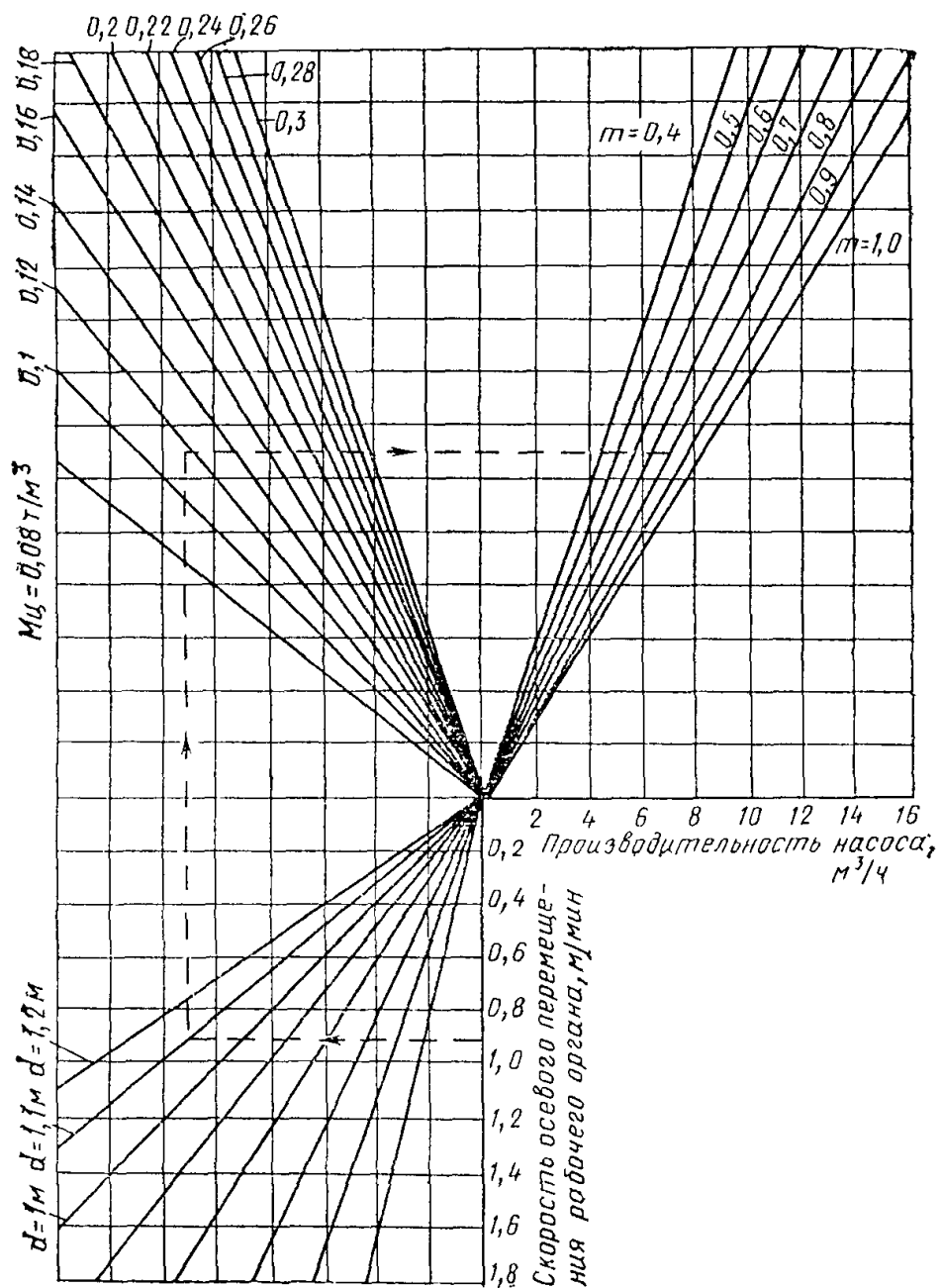
Номограмма для определения производительности насоса в зависимости от скорости осевого перемещения буросмесителя, диаметра сваи ( d ), дозировки цемента ( M_{ц} ) и водоцементного отношения ( m )
