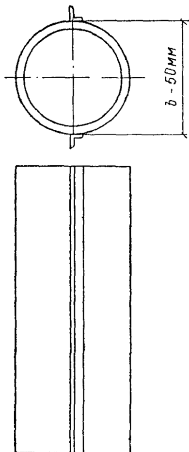
Рис. 81. Трубчатый ограничитель
