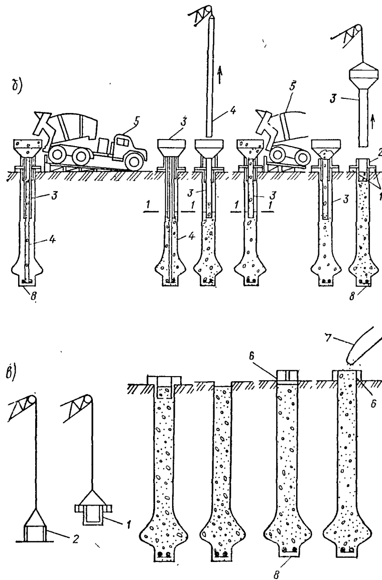
Рис. 8. Бетонирование скважин для свай методом ВПТ
