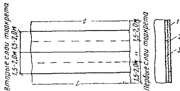
Рис. 92. Порядок нанесения слоев торкрет-гидроизоляции
