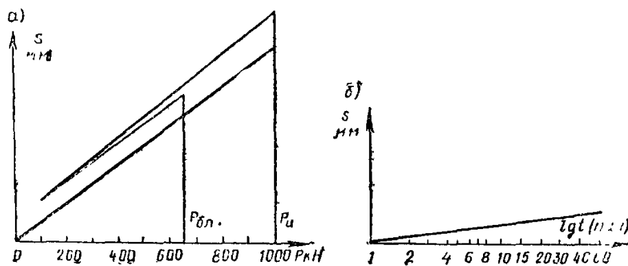
Рис. 2. Приемочные испытания анкеров
