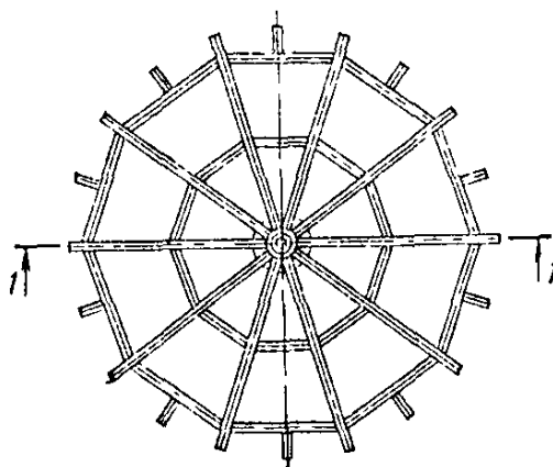
Рис. 97. Кондуктор стационарного типа
