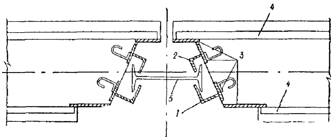
Рис. 84. Съёмная (инвентарная) направляющая
