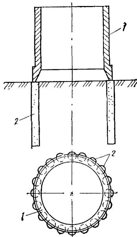
Рис. 89. Схема закрепления основных осей опускного колодца или кессона на местности
