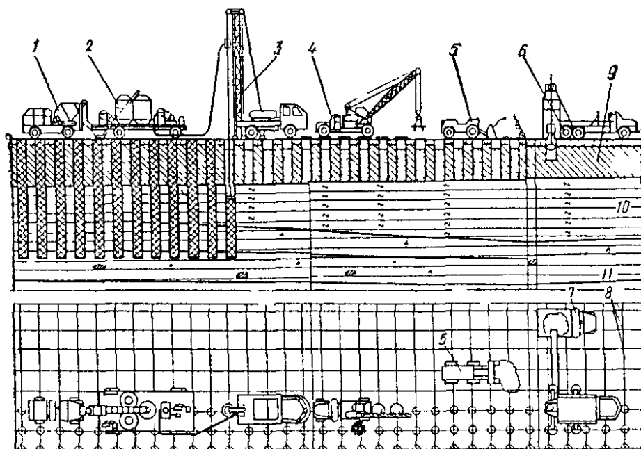
Рис. 1. Укрепление основания буромесительным способом с использованием серийной буровой установки с работающим в непосредственной близости от нее растворонасосным узлом, смонтированным на передвижном шасси
