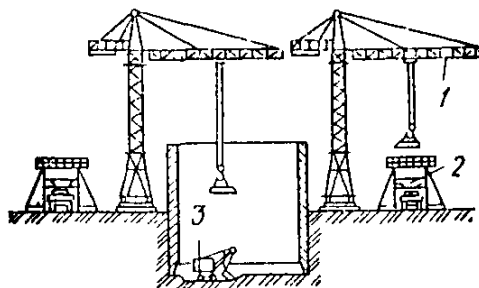
Рис. 104. Разработка грунта экскаватором
