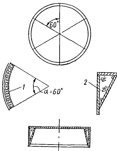
Рис. 108. Ножевая часть опускного колодца
