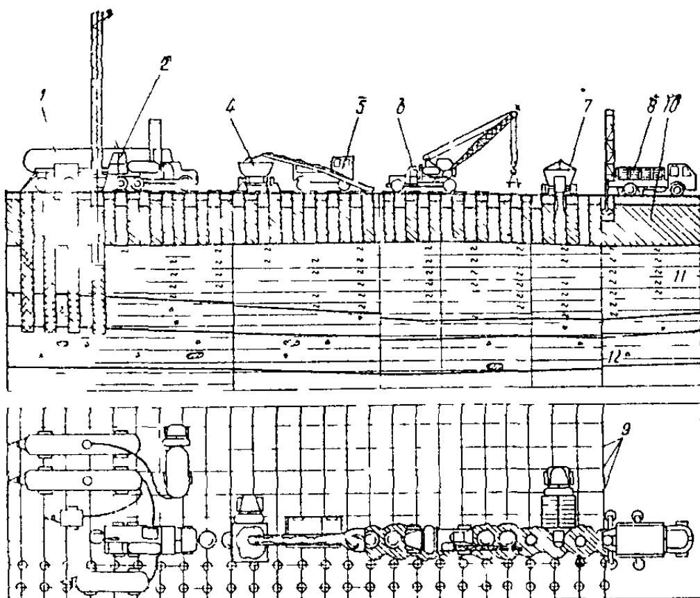
Рис. 2. Укрепление основания буромесительным способом с использованием серийной буровой установки с передвижным растворонасосным узлом с центральной буровой установки с передвижным растворонасосным узлом снабжаемым цементным раствором с центрального бетонорастворного узла
