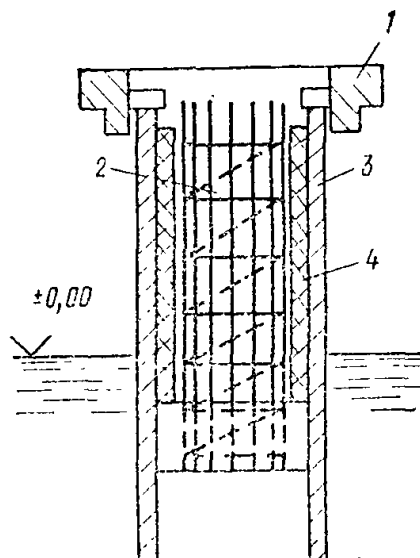
Рис. 6. Схема устройства амортизирующего слоя на свая-оболочке
