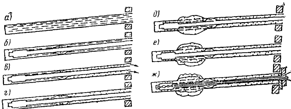
Рис. 4. Технология устройства анкера с манжетной трубой при внутреннем расположении тяги с двухкратной иньекцией
